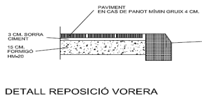
DETALL REPOSICIÓ VORERA
