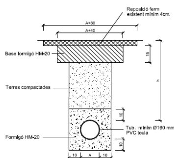
SECCIÓ A-A'
